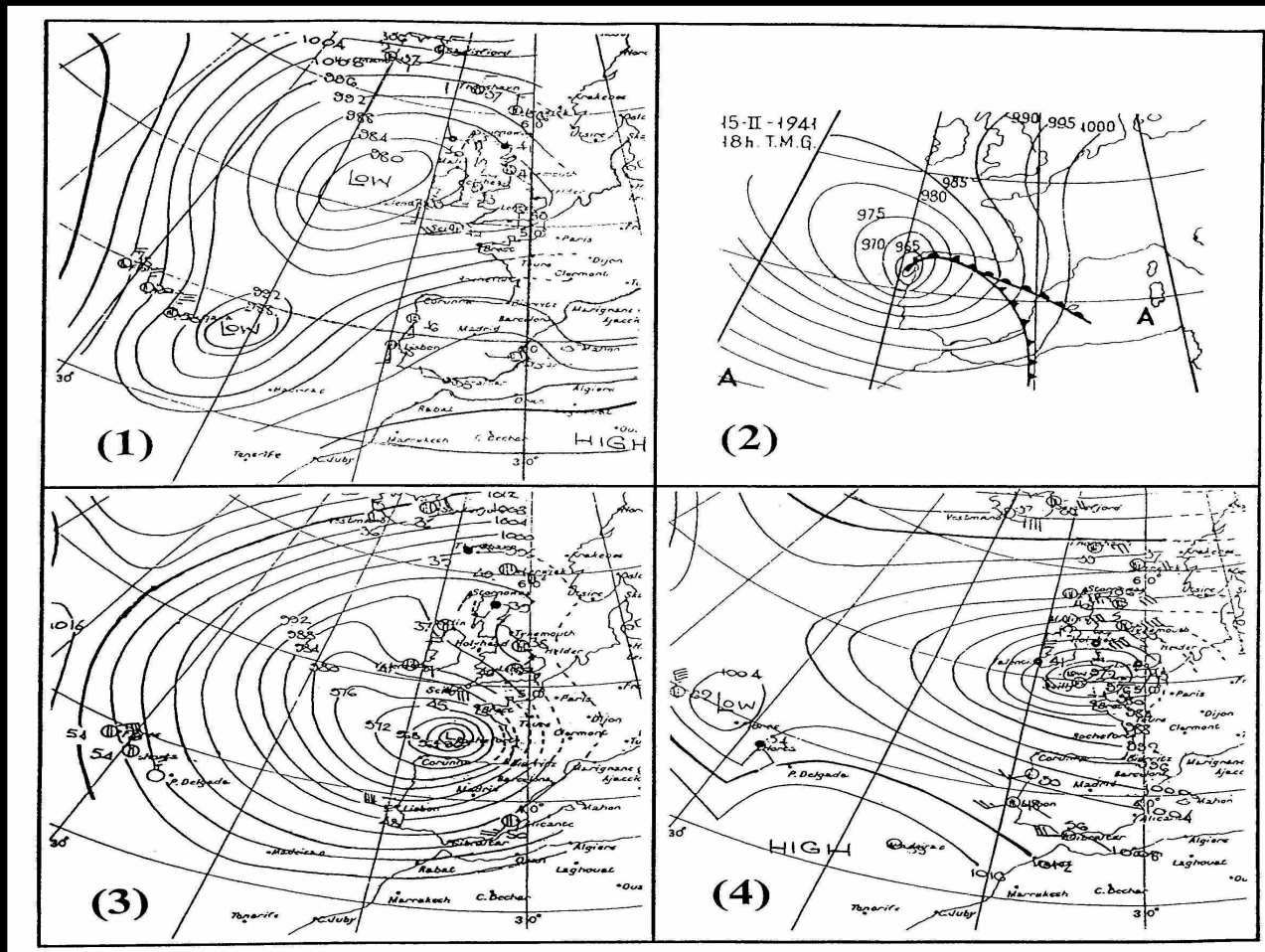
FIGURA 2.-Evolución atmosférica en superficie durante el temporal de febrero de 1941. FUENTE: mapas 1, 3 y 4: Met Office; mapa 2: Mateo González, P.(1955).
