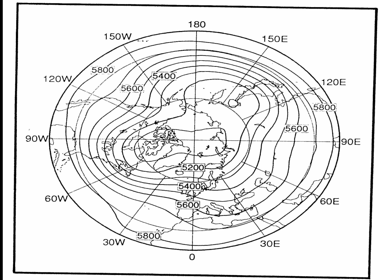
FIGURA 1.-Mapa promedio de las isohipsas correspondientes al nivel de 500 hPa para el Hemisferio Norte durante el mes de enero. FUENTE: Hartmann, D. L. en Global Physical Climatology (1994).
